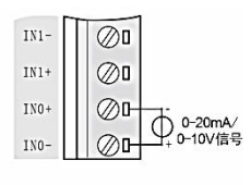
模块输入信号接线图
