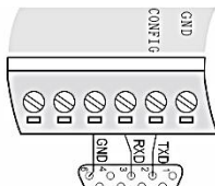
RS232接口
