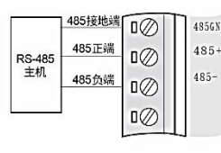
RS485接口接线图
