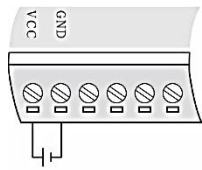
电源:4-50VDC
