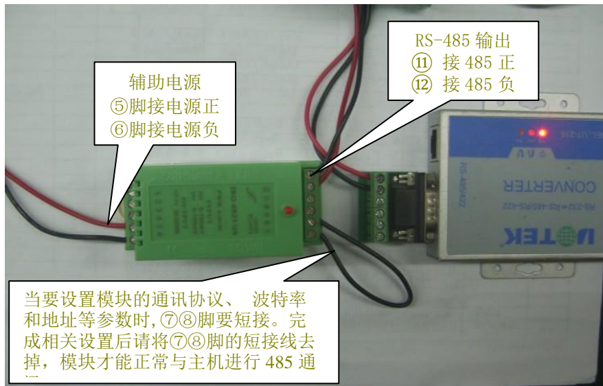
图中: ISO4021 的 5 脚和 6 脚外接电源为 8-50V, 当通讯接口选型为 RS485 时, RS485 的信号正端和负端分别接产品的 DATA+,DATA-接口, 并且 RS232 和 RS485 不能同时工作。第 8 脚是配置端口 CONFIG, 设置通讯协议时请将 CONFIG 脚与 7 脚地连接起来。
