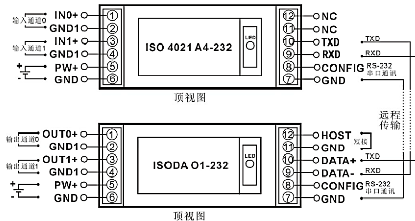
ISO 4021 与 ISO DA 的 RS232 通讯方式接线图
